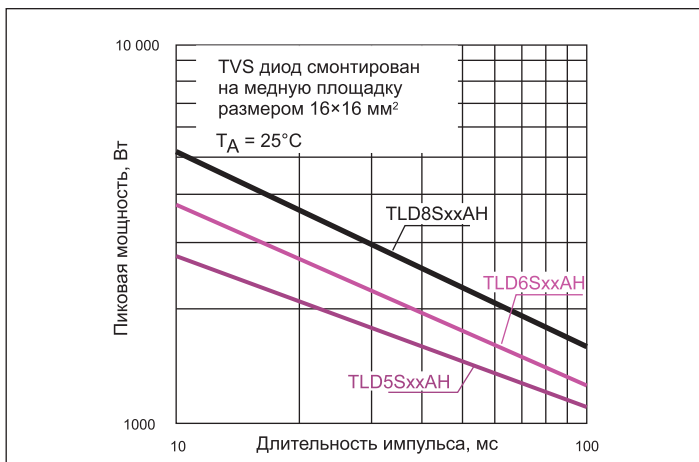
Рис. 4. Зависимость пиковой мощности TVS от длительности импульса
