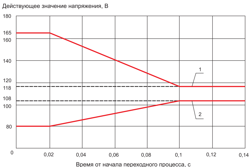
Рис. 5. Требования ГОСТ Р 54073-2010 к переходным напряжениям
