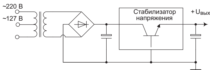
Рис. 23. «Трансформаторный» ИВЭП
