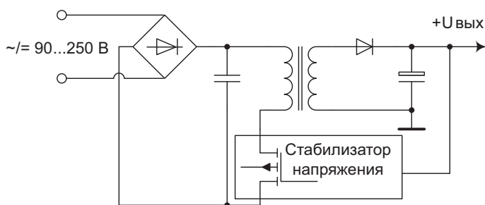
Рис. 24. «Бестрансформаторный» ИВЭП с высоким КМ
