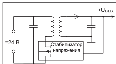
Рис. 25. ИВЭП для низковольтной DC-сети
