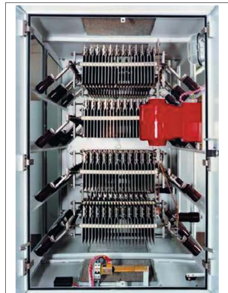
Рис. 7. Заземляющий резистивный модуль TERA
